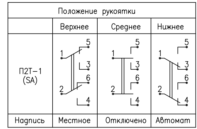
Диаграмма замыкания контактов переключателей
